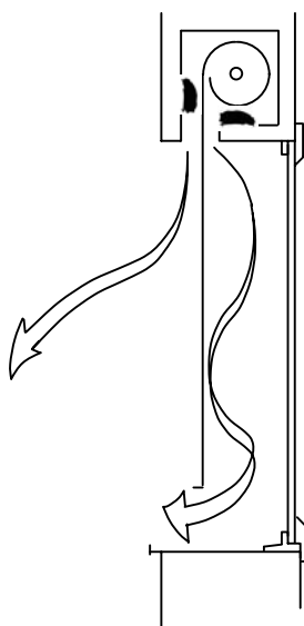
Figure 3 : Stores pas complètement descendus, fenêtre fermée : solution sûre.
