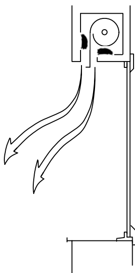
Figure 2 : Stores remontés, fenêtre fermée : la solution la plus sûre.
